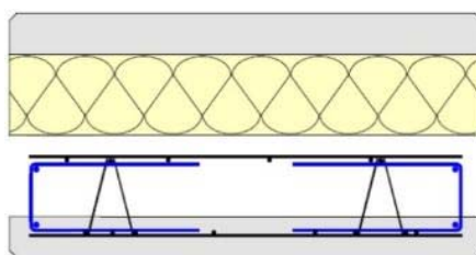
Figure 84 - Cadres + épingles
