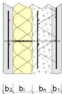
Figure 42 - Section et épaisseurs d'un « Duomur Isolant »
