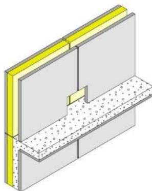
Figure 41 - Détail de réalisation du fractionnement des acrotères hauts
