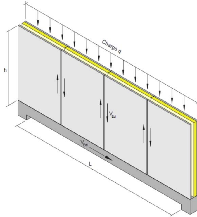
Figure 53 - Effort sollicitant dans le cas d'une poutre-voile
