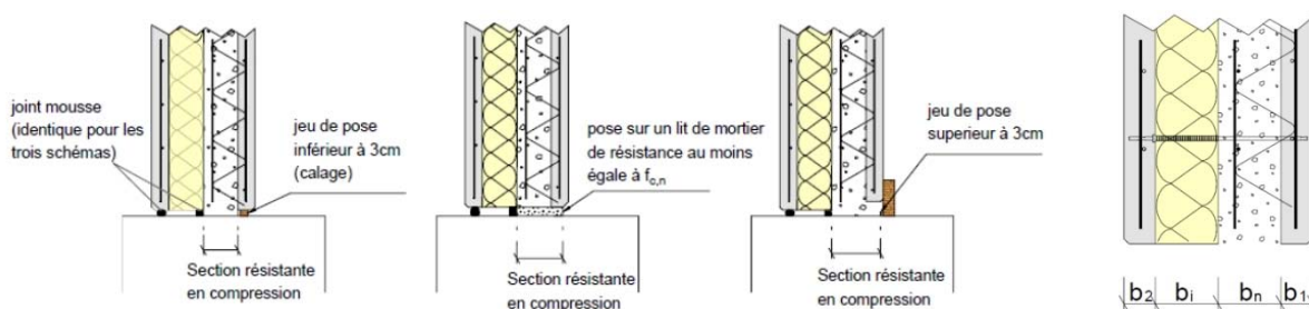
Figure 14 - Exemple de section résistante en compression
