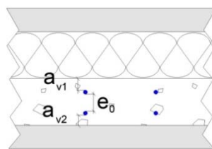
Figure 24 - Exemple de l'éclissage des armatures verticales
