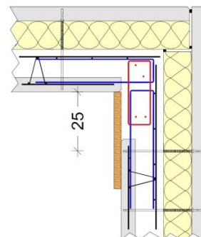
Figure 111 - Coffrage de la face intérieure, avec ou sans aciers en attente
