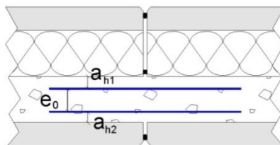
Figure 23 - Exemple de l'éclissage des armatures horizontales
