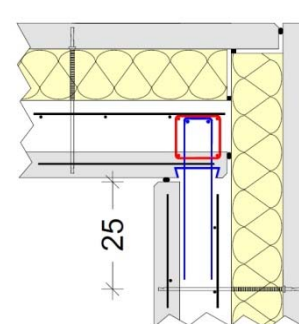
Figure 108 - Liaison par boîte d'attente
