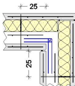
Figure 104 - 2 lits d'armatures de liaison
