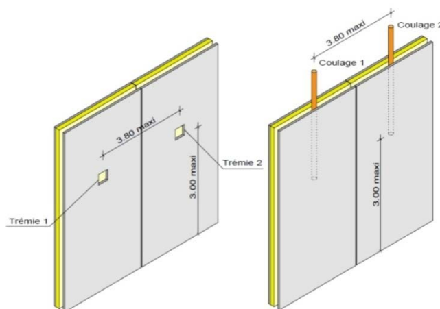
Figure 25 - Hauteur de bétonnage équivalente à (a) hauteur sous trémie et (b) hauteur sous tube souple
