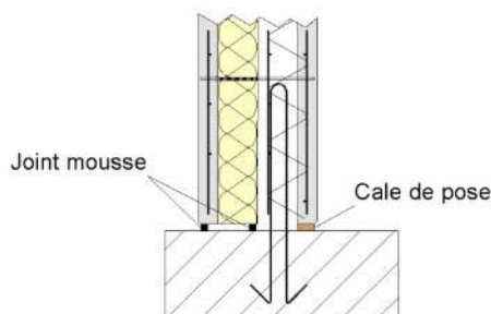
Figure 30 - Liaisons en pied de murs courants
