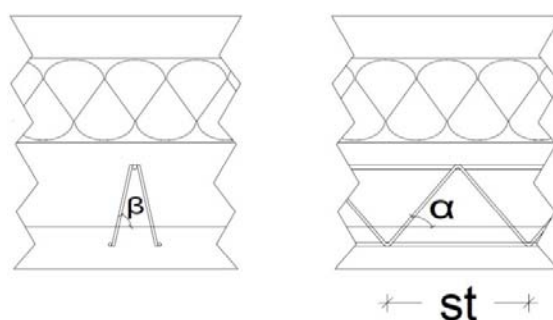
Figure 20 - Géométrie du raidisseur
