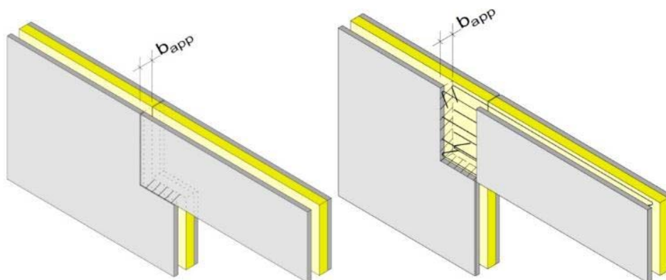
Figure 36 - Appui de poutre – cas 2
