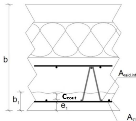
Figure 17 - Définition des chaînes de cotes
