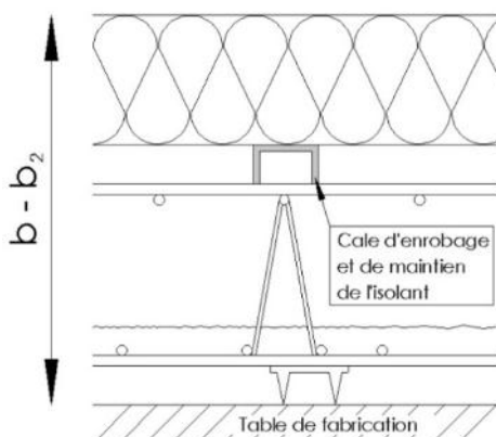
Figure 10 – Cale d'enrobage contre l'isolant
