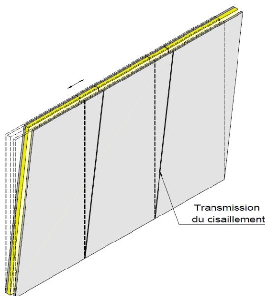
Figure 26 - Schéma d'un comportement monolithique des panneaux
