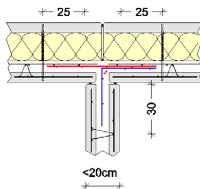
Figure 113 - 1 + 1 lit d'armatures, parois décroisées
