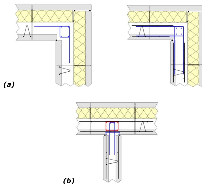
Figure 28 - Exemple d'intersections de mur
