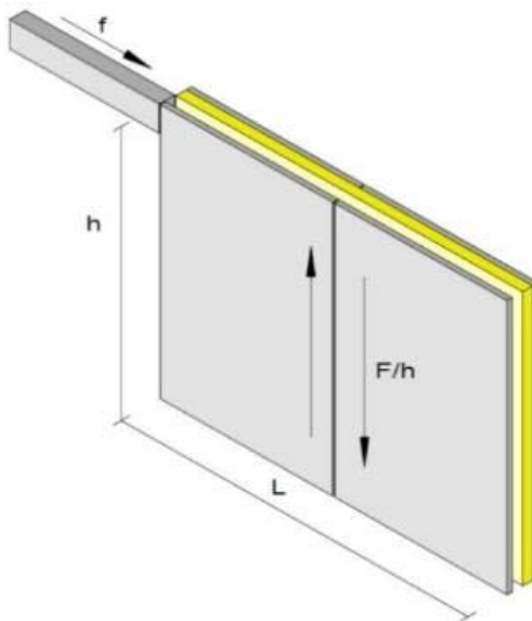
Figure 52 (a) – Effort sollicitant dans le cas d'une charge ponctuelle
