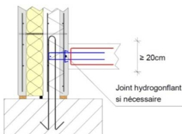
Figure 86 - 2 lits d'armatures en attente
