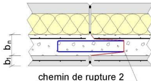
Figure 55 – Liaison sans coutures aux abouts
