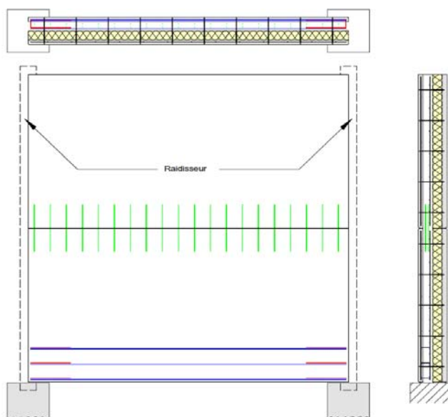
Figure 60 – Poutre voile réalisé en plusieurs « Duomur Isolant » superposés
