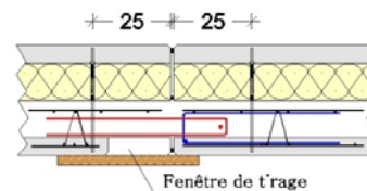
Figure 100 - Liaison couturée
