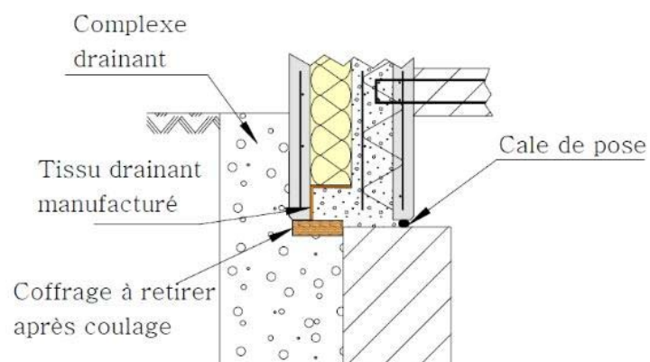
Figure 68 – Détail sur tissu drainant manufacturé
