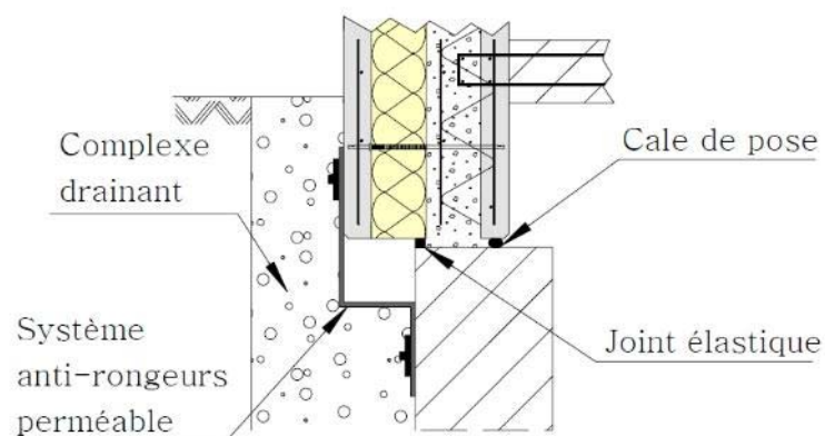
Figure 67 – Pied de murs protégé par le béton de remplissage
