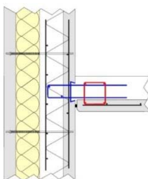
Figure 94 - Plancher suspendu avec boîte d'attente. Celles-ci doivent respecter les dispositions de l'annexe F de la section A du « Cahier 2892_V3 (mai 2020) ou celles du NF DTU 23.4 à compter de sa parution en remplacement du Cahier 2892_V2 »
