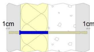
Figure 9 – Enrobage nominal des connecteurs
