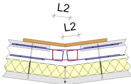
Figure 110 - Angles > à 165° L2 = 32 \varnothing + 7 \text{ cm}
