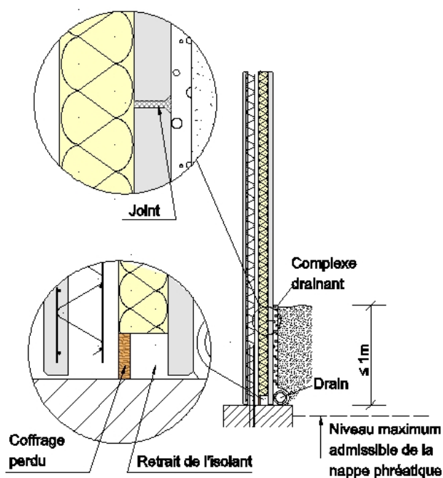
Figure 43 – Murs semi enterrés faible hauteur
