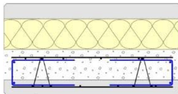
Figure 31 - Section de poteau résistant par le béton seul
