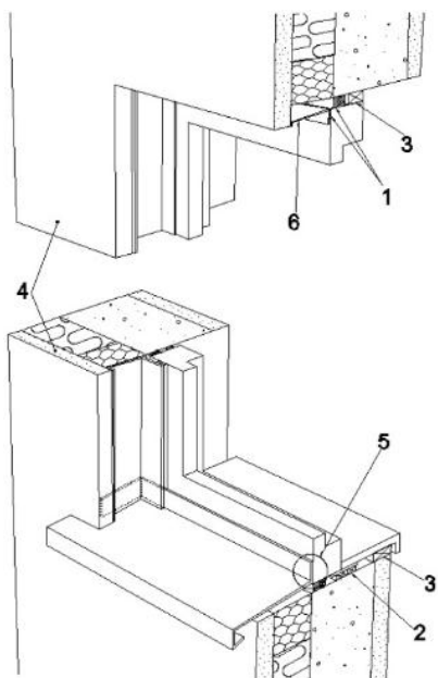
Figure 48 – Exemple de menuiserie à l'interface isolant/béton de remplissage
