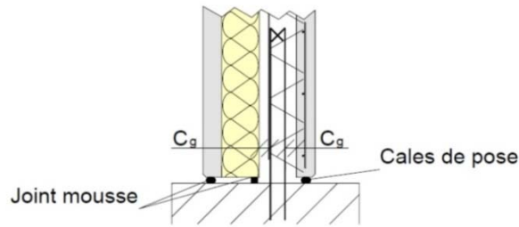
Figure 22 - Position des aciers en attente dans un « Duomur Isolant »
