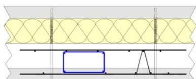
Figure 74 - Poteau intégré au « Duomur Isolant »
