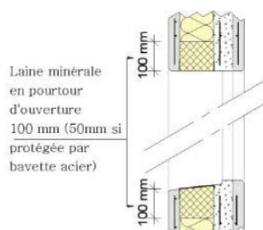
Figure 46 – Laine minérale en pourtour d'ouverture
