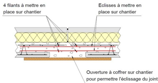
Figure 27 - Liaison verticale en zone sismique sans justification par le calcul
