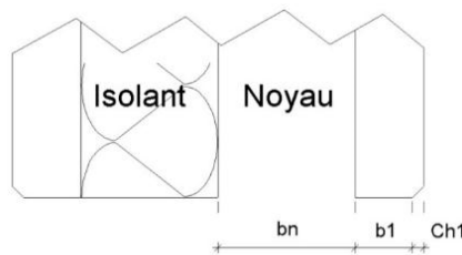
Figure 34 – Définition de géométrie de la section
