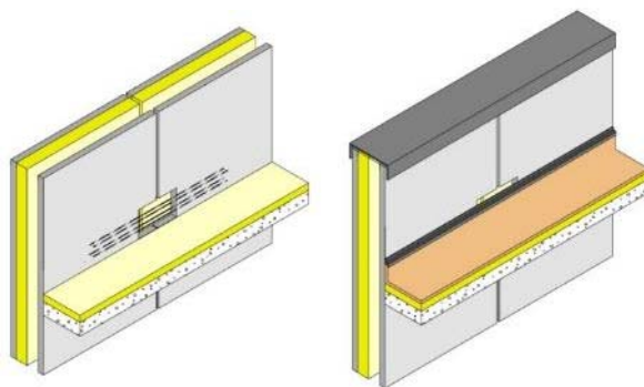
Figure 40 - Acrotères hauts réalisés par des pièces complémentaires au-dessus de la toiture
