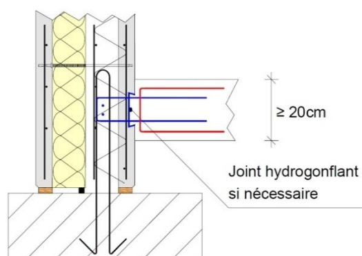
Figure 92 - Liaison encastrée avec un plancher bas
