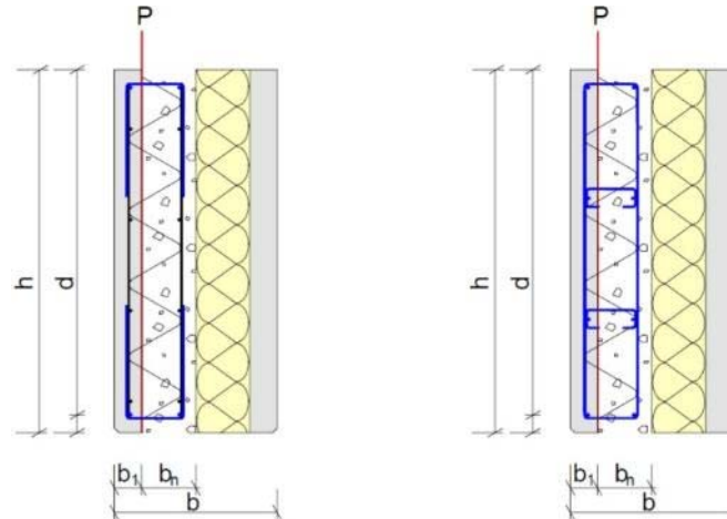
Figure 33 - Plans de cisaillement dans la section d'une poutre
