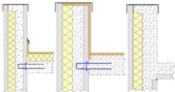
Figure 37 - Protection de l'étanchéité
