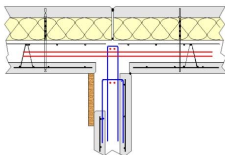
Figure 121 - Joint au droit du refend sans aciers en attente
