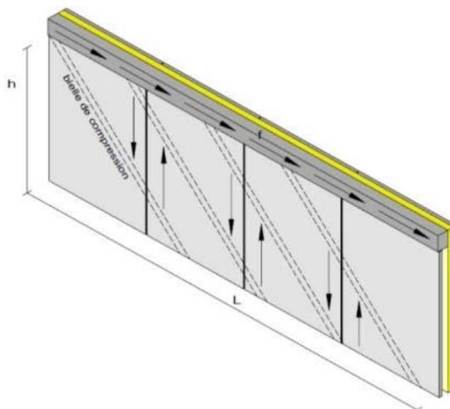
Figure 52 (b) – Effort sollicitant dans le cas d'une charge linéaire horizontale
