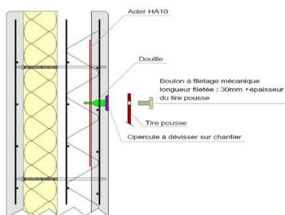
Figure 73 - Détail sur douille d'étaie
