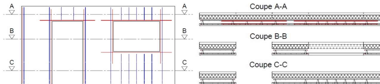
Figure 19 - Dispositions équivalentes de renforcement des bords libres verticaux solution « Duomur Isolant »
