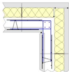
Figure 109 - « Duomur Isolant » » posé avant réalisation du support
