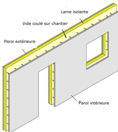
Figure 2 – Exemple d'élément « Duomur Isolant »
