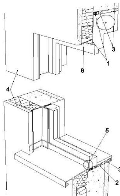
Figure 50 – Exemple de mise en place de volet roulant
