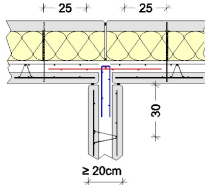
Figure 115 - 1 + 2 lits d'armatures, parois décroisées
