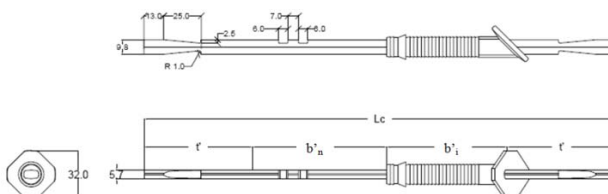
Figure 7 - Détail d'un connecteur TM45°
