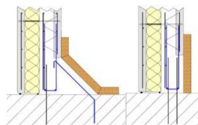
Figure 90 - Coffrage d'une face sur chantier
