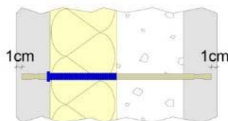
Figure 15 - Retrait minimum des connecteurs : 1 cm
