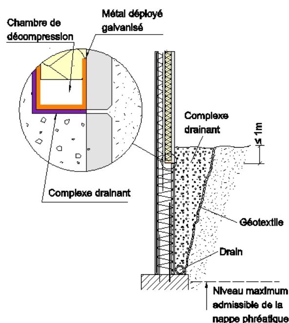
Figure 44 – Murs semi enterrés hauteur importante
