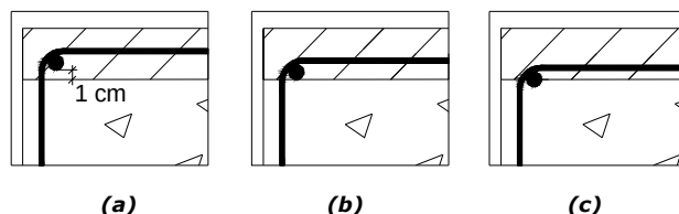
Figure 21 - Enrobage des aciers structuraux et périmètre utile
