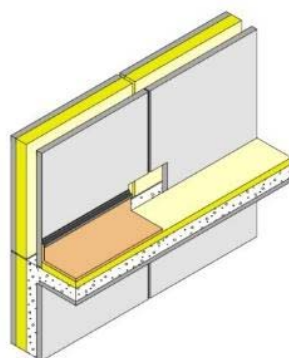
Figure 41 - Détail de réalisation du fractionnement des acrotères hauts
