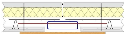
Figure 76 - Poteau coulé en place au droit d'un joint vertical – Coffrage d'une face
