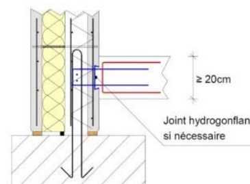
Figure 87 - Liaison couturée avec plancher bas
