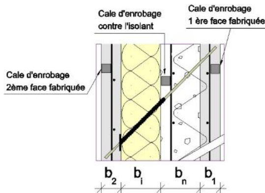
Figure 8 - Positionnement des connecteurs à 45°
