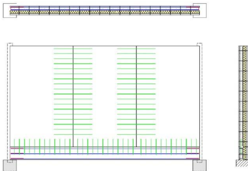
Figure 61 – Poutre voile en plusieurs parties
