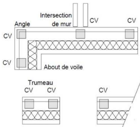
Figure 29 - Implantation type des chaînages verticaux CV
