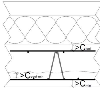
Figure 16 - Définition des enrobages
