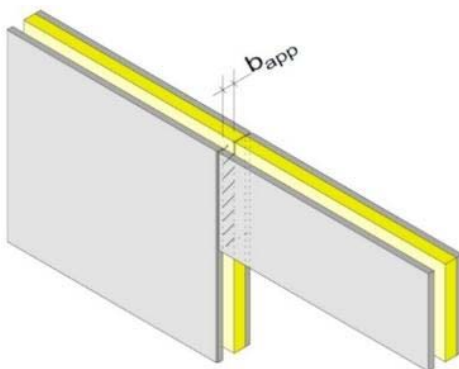
Figure 35 - Appui de poutre – cas 1
