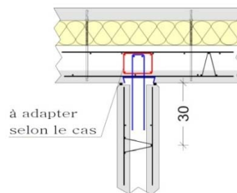
Figure 118 - Liaison par boîte d'attente
