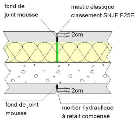
Figure 64 - Traitement des joints entre « Duomur Isolant »
