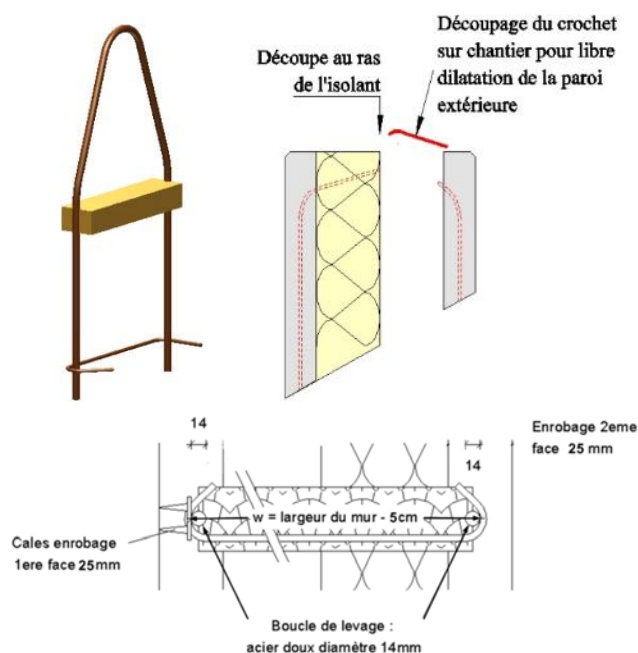
Figure 3 : Boucle de levage pour « Duomur Isolant »
