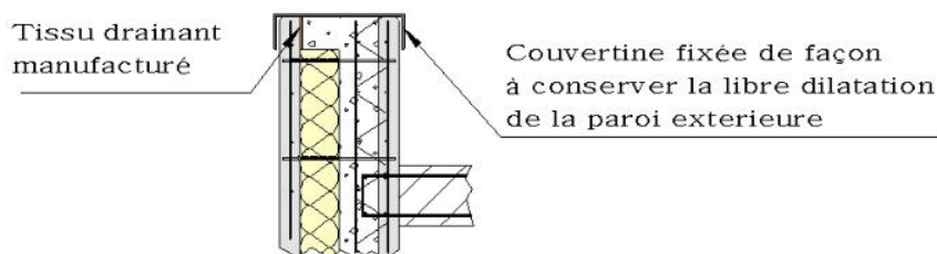
Figure 67 – Pied de mur protégé par système anti-rongeur
