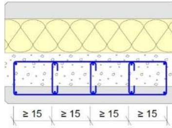
Figure 32 - Section de poteau nécessitant des armatures structurales
