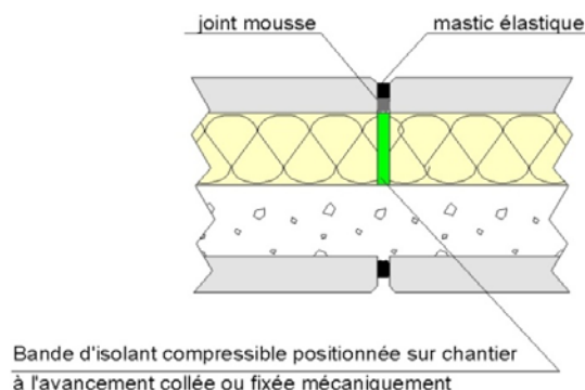
Figure 45 - Jonction entre épaisseurs isolantes
