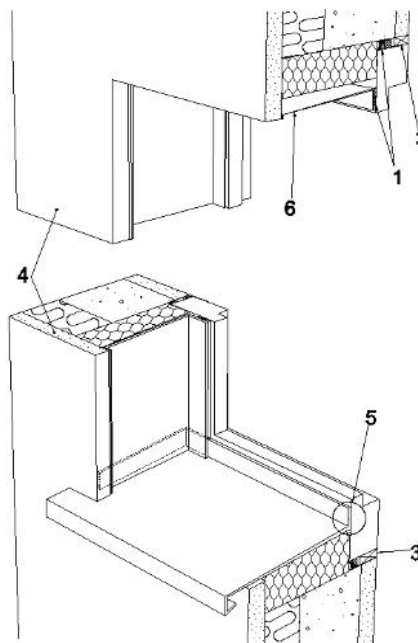
Figure 49 – Exemple de menuiserie au nu intérieur du « Duomur Isolant »
